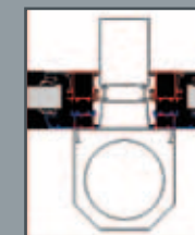
obudowa spływu 180°
