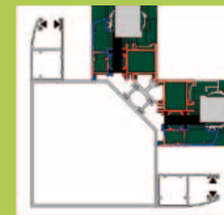
słup equinoxe do mocowania prowadnic
