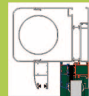
słup equinoxe ze spływem wody
